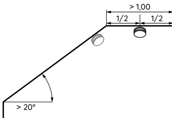
Abb. 5 Gerade Montagefläche mindestens 1 m lang und 1 m breit
